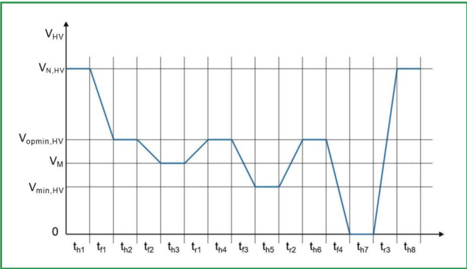
EHV-03 高压欠压范围内的高压电压曲线
